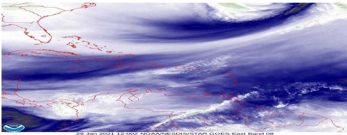
Figura 5: Imagen satelital GOES vapor de agua, enero 29 de 2021, hora 7:00 am de Colombia. Fuente: NOAA.
