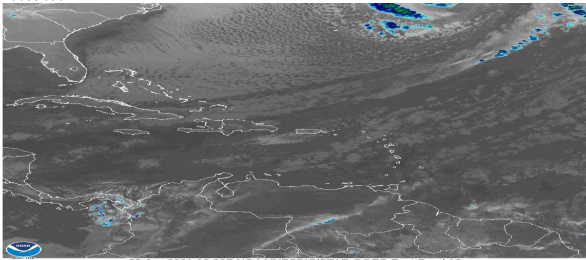
Figura 4: Imagen satelital GOES, enero 29 de 2021, hora 7:00 am de Colombia. Fuente: NOAA.
