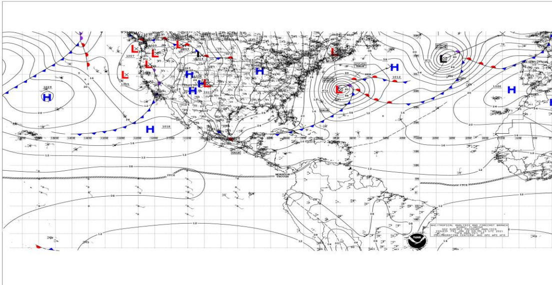
Figura 1: Situación meteorológica actual en el Mar Caribe y Océano Atlántico, enero 29 de 2021, Fuente: NHC NOAA.
