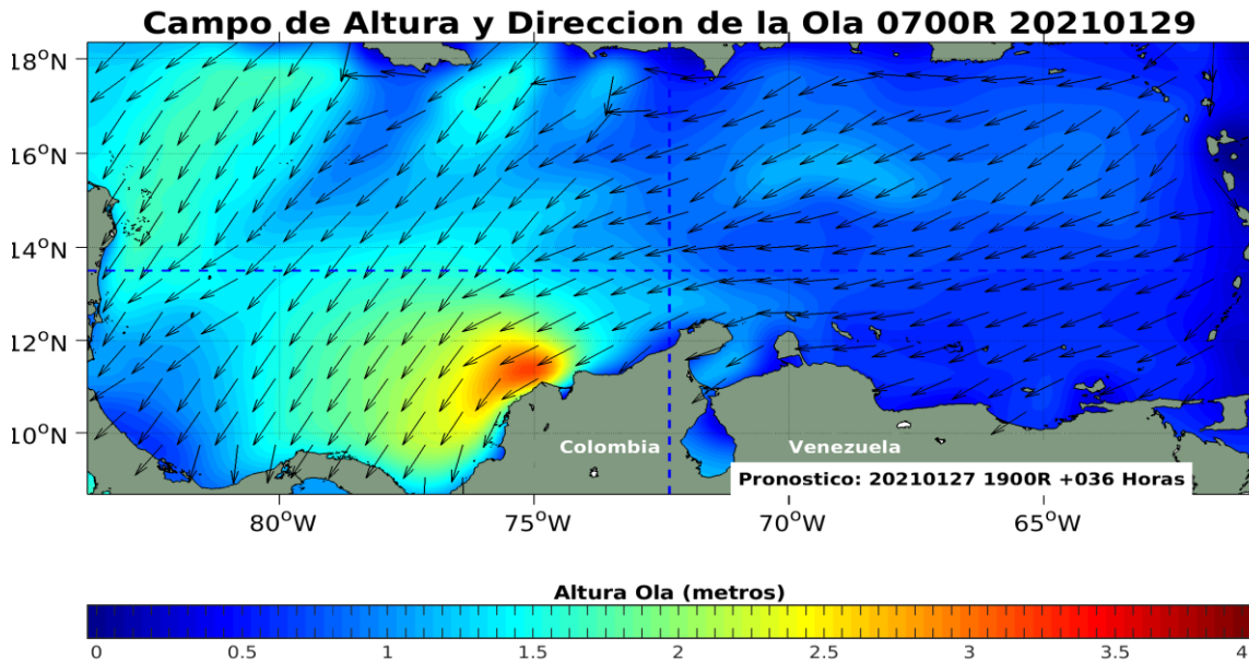
Figura 6: Pronóstico de la altura y dirección de las olas en el Mar Caribe, enero 29 de 2021. Fuente: CIOH.
