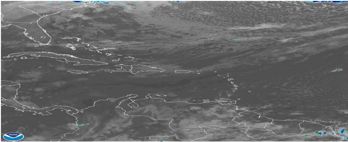
Figura 4: Imagen satelital GOES, enero 31 de 2021, hora 7:00 am de Colombia. Fuente: NOAA
