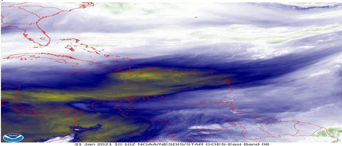
Figura 5: Imagen satelital GOES vapor de agua, enero 31 de 2021, hora 7:00 am de Colombia. Fuente: NOAA.
