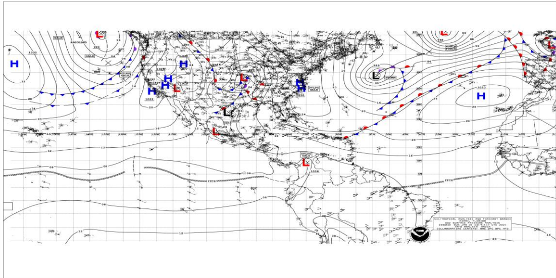
Figura 1: Situación meteorológica actual en el Mar Caribe y Océano Atlántico, enero 31 de 2021, Fuente: NHC NOAA.
