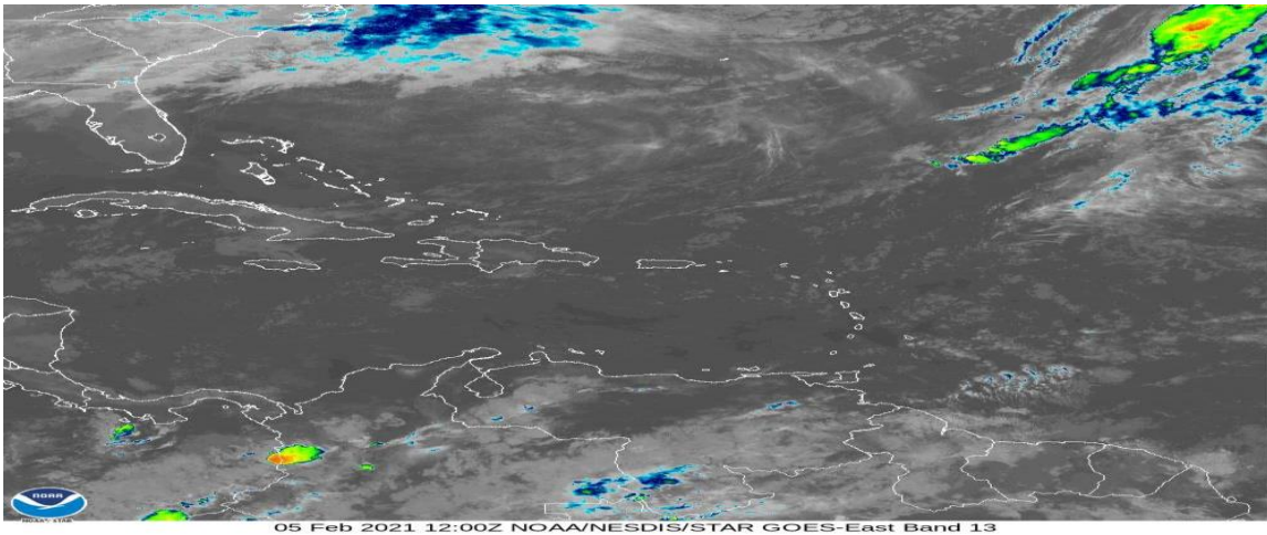
Figura 4: Imagen satelital GOES, febrero 5 de 2021, hora 7:00 am de Colombia. Fuente: NOAA
