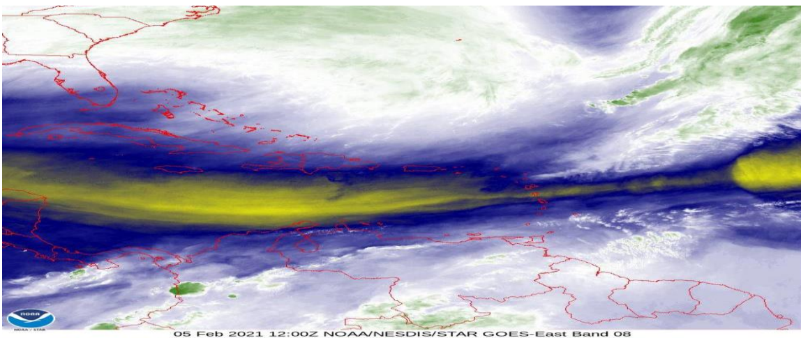
Figura 5: Imagen satelital GOES vapor de agua, febrero 5 de 2021, hora 7:00 am de Colombia. Fuente: NOAA.
