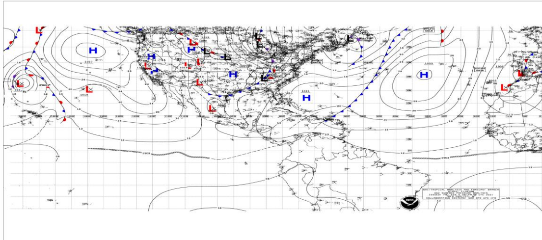
Figura 1: Situación meteorológica actual en el Mar Caribe y Océano Atlántico, febrero 5 de 2021, Fuente: NHC NOAA.
