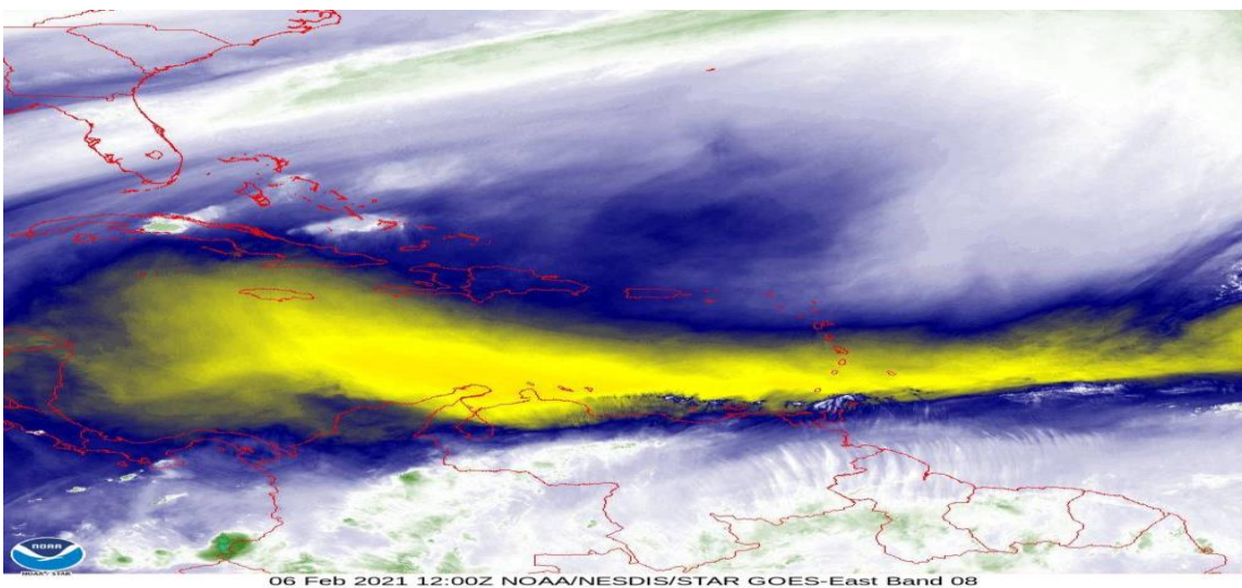
Figura 5: Imagen satelital GOES vapor de agua, febrero 6 de 2021, hora 7:00 am de Colombia. Fuente: NOAA.
