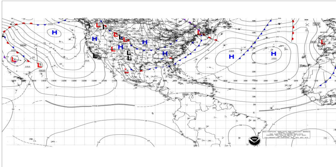
Figura 1: Situación meteorológica actual en el Mar Caribe y Océano Atlántico, febrero 6 de 2021, Fuente: NHC NOAA.
