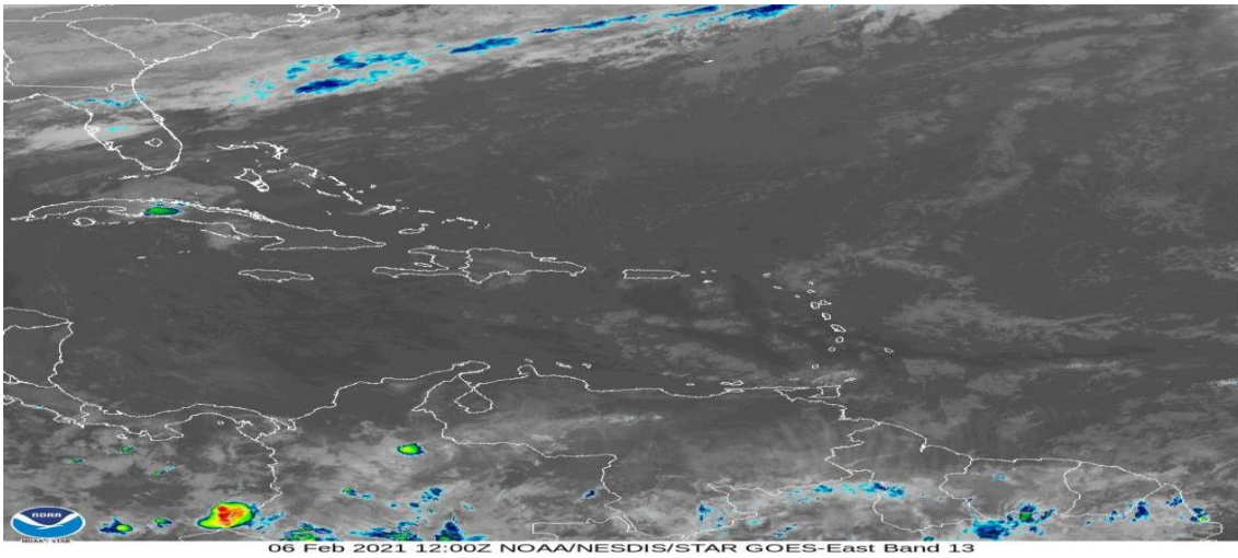
Figura 4: Imagen satelital GOES, febrero 6 de 2021, hora 7:00 am de Colombia. Fuente: NOAA
