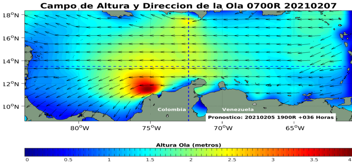
Figura 6: Pronóstico de la altura y dirección de las olas en el Mar Caribe, febrero 6 de 2021. Fuente: CIOH.
