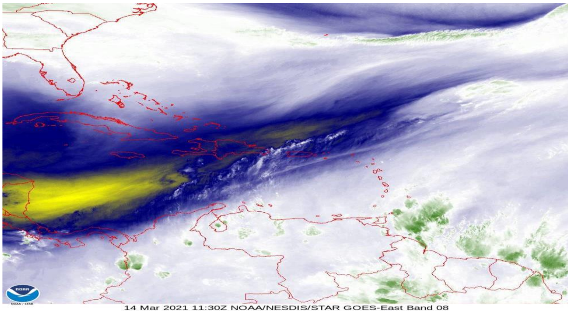
Figura 2: Imagen satelital de vapor de agua generada por el satélite Geoestacionario GOES de la NOAA, para el día 14 de marzo de 2021, hora 06:30 HLC, se utiliza principalmente para determinar los sitios secos (color amarillo y negro) y húmedos (color azul, blanco, verde); como muestra la figura, actualmente se presenta abundante humedad en gran parte del territorio de La Guajira y principalmente en el centro y el sur, que puede generar lluvias y lloviznas sectorizadas.
