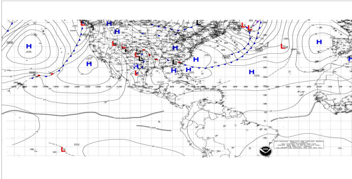
Figura 1: Muestra la situación meteorológica en superficie en el Mar Caribe y Océano Atlántico, para el día 14 de marzo de 2021 a las 03:35 HLC, se muestra principalmente los centros de alta (H) y baja (L) presión atmosférica, la fuente de la información es el Centro Nacional de Huracanes NHC de Miami que hace parte de la Administración Nacional del Océano y la Atmósfera NOAA.
