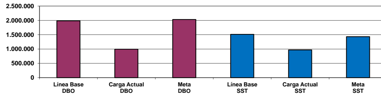
Grafica 1. Comportamiento de las Cargas Contaminantes (kg/año)
