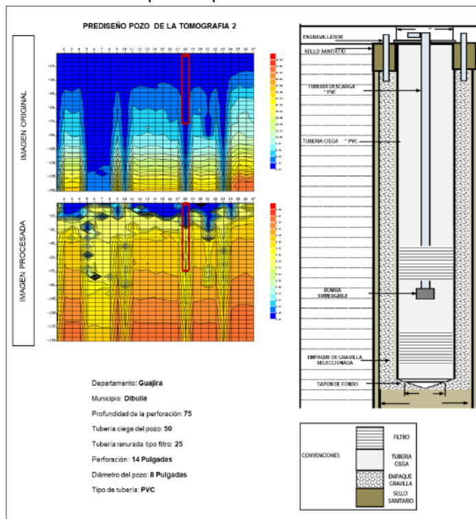
Grafica 3. Prediseño del pozo exploratorio de conformidad a los resultados
