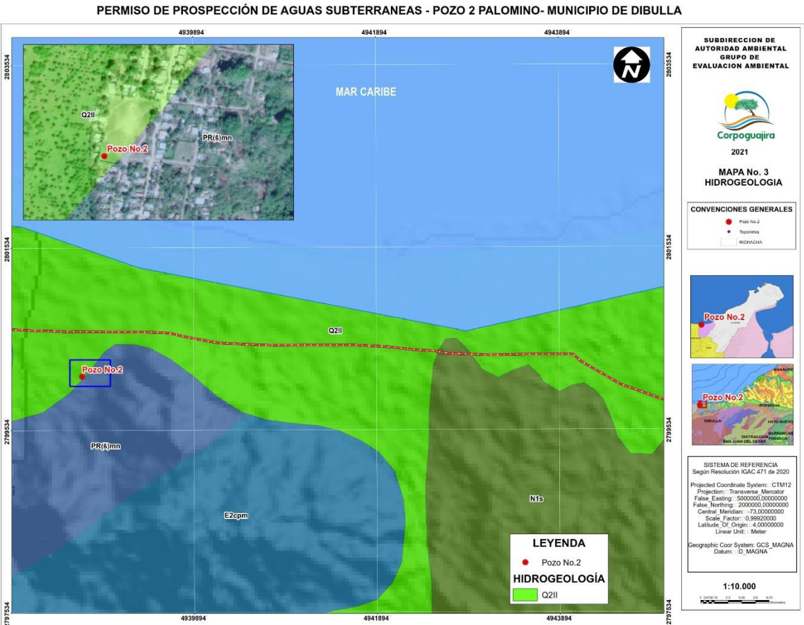
Figura 4. Hidrogeología del área del estudio según estudio realizado por el SGC en el departamento de La Guajira.
