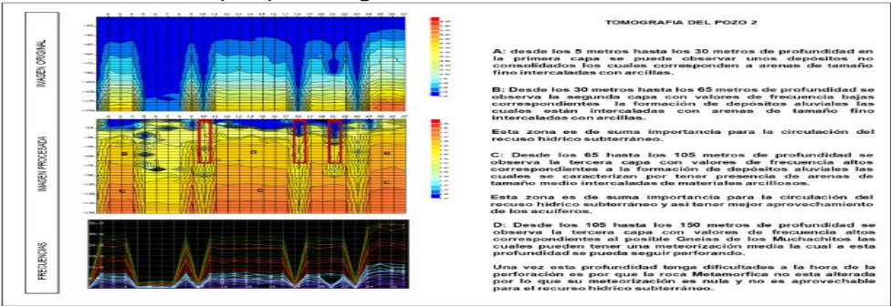
Grafica 3. Metodología Resultados y modelo de capas del pozo: fuente tomada de aplicación de método eléctrico de prospección geofísica TOM-2
