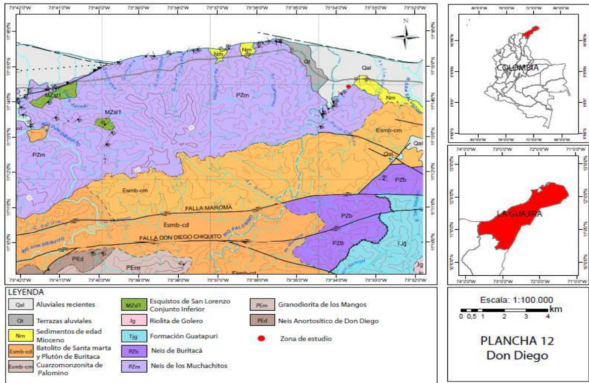
Figura 3. Mapa Geológico Regional. Plancha 12 Don Diego Servicio Geológico Colombiano.
