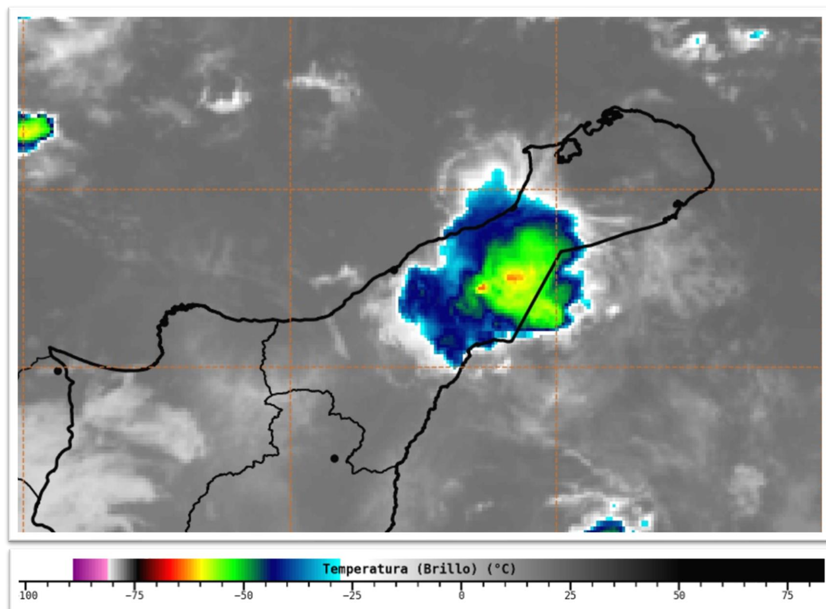
Imagen satelital Infrarojo GOES 16 Septiembre 06 de 2021 – Hora 7:10 HLC. Fuente: IDEAM
