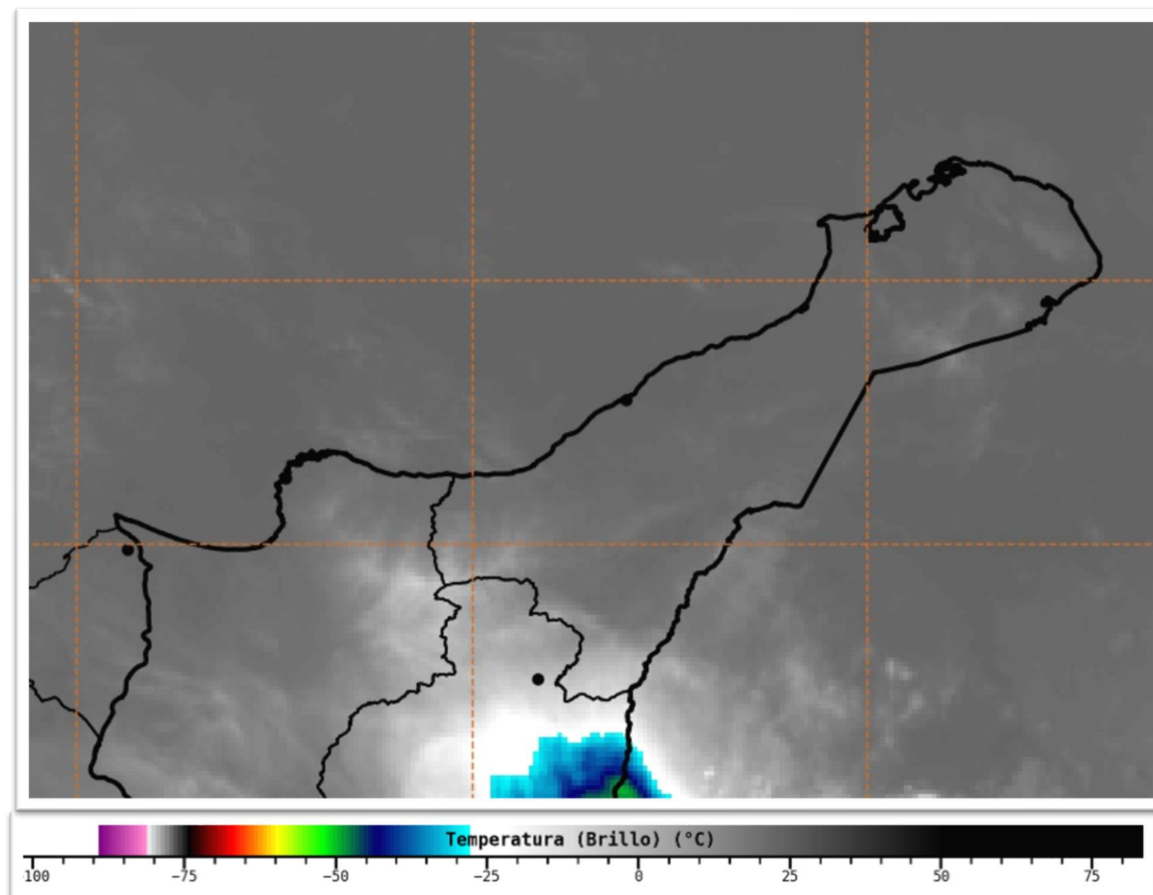
Imagen satelital Infrarojo GOES 16 Septiembre 09 de 2021 – Hora 7:00 HLC. Fuente: IDEAM
