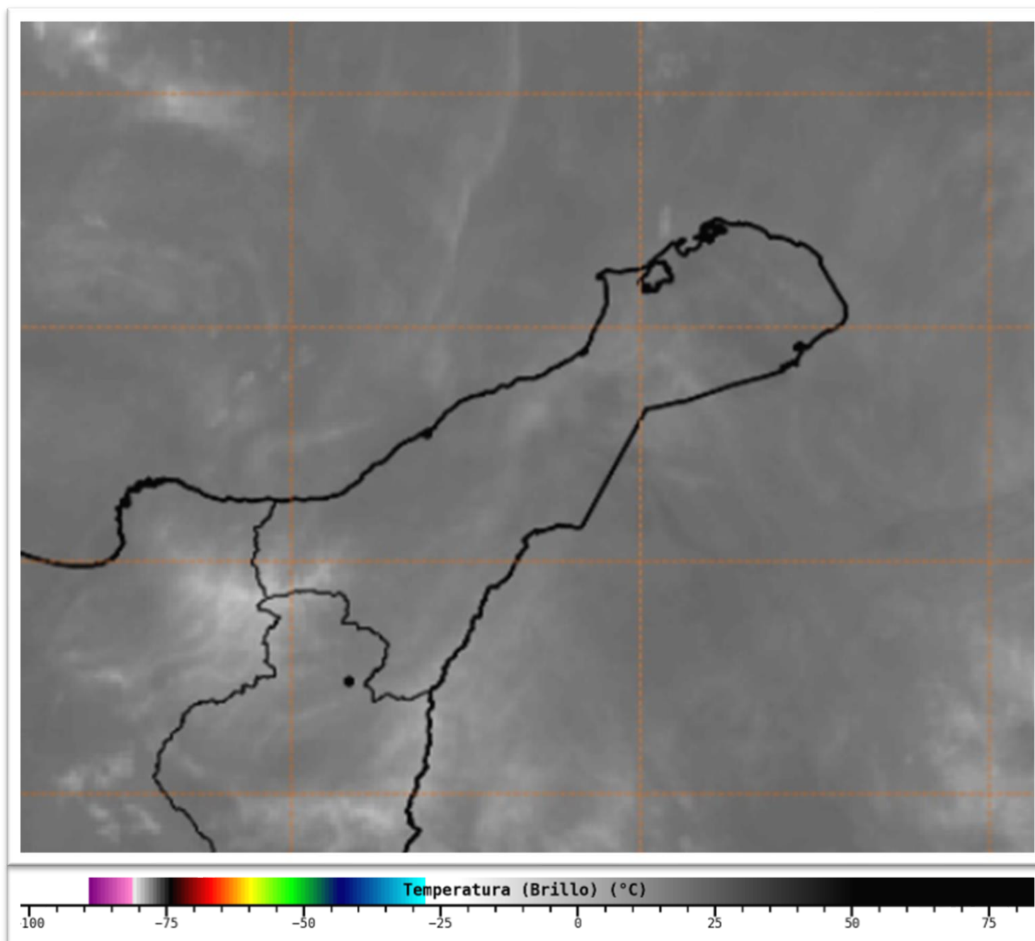
Imagen satelital Infrarojo GOES 16 Agosto 12 de 2021 – Hora 7:20 HLC. Fuente: IDEAM
