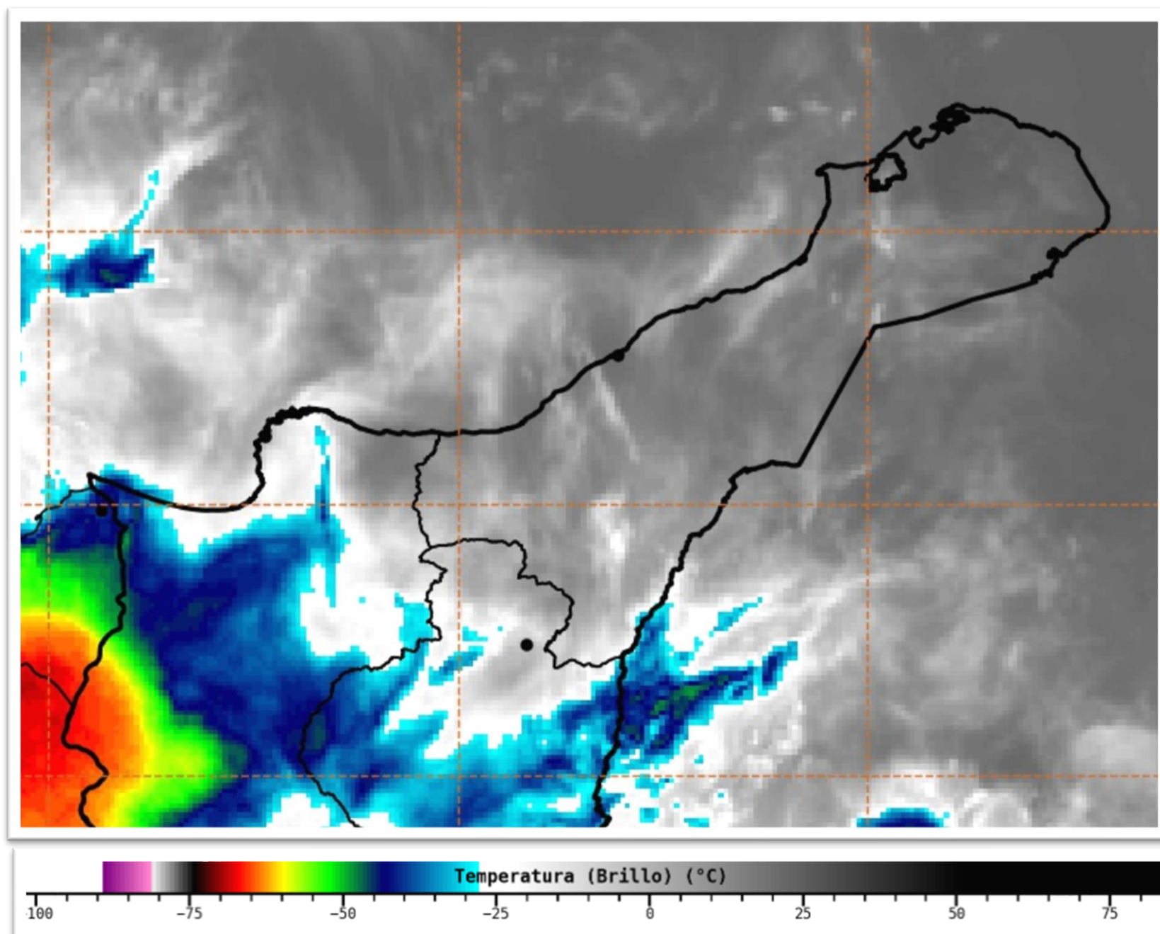
Imagen satelital Infrarojo GOES 16 Septiembre 16 de 2021 – Hora 7:10 HLC. Fuente: IDEAM
