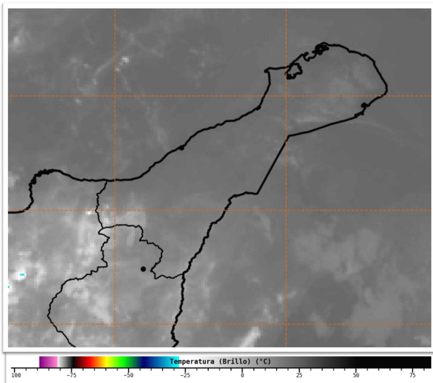
Imagen satelital Infrarojo GOES 16 Agosto 17 de 2021 – Hora 7:00 HLC. Fuente: IDEAM
