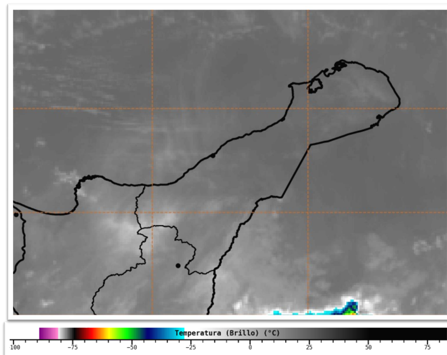
Imagen satelital Infrarojo GOES 16 Agosto 19 de 2021 – Hora 6:50 HLC. Fuente: IDEAM
