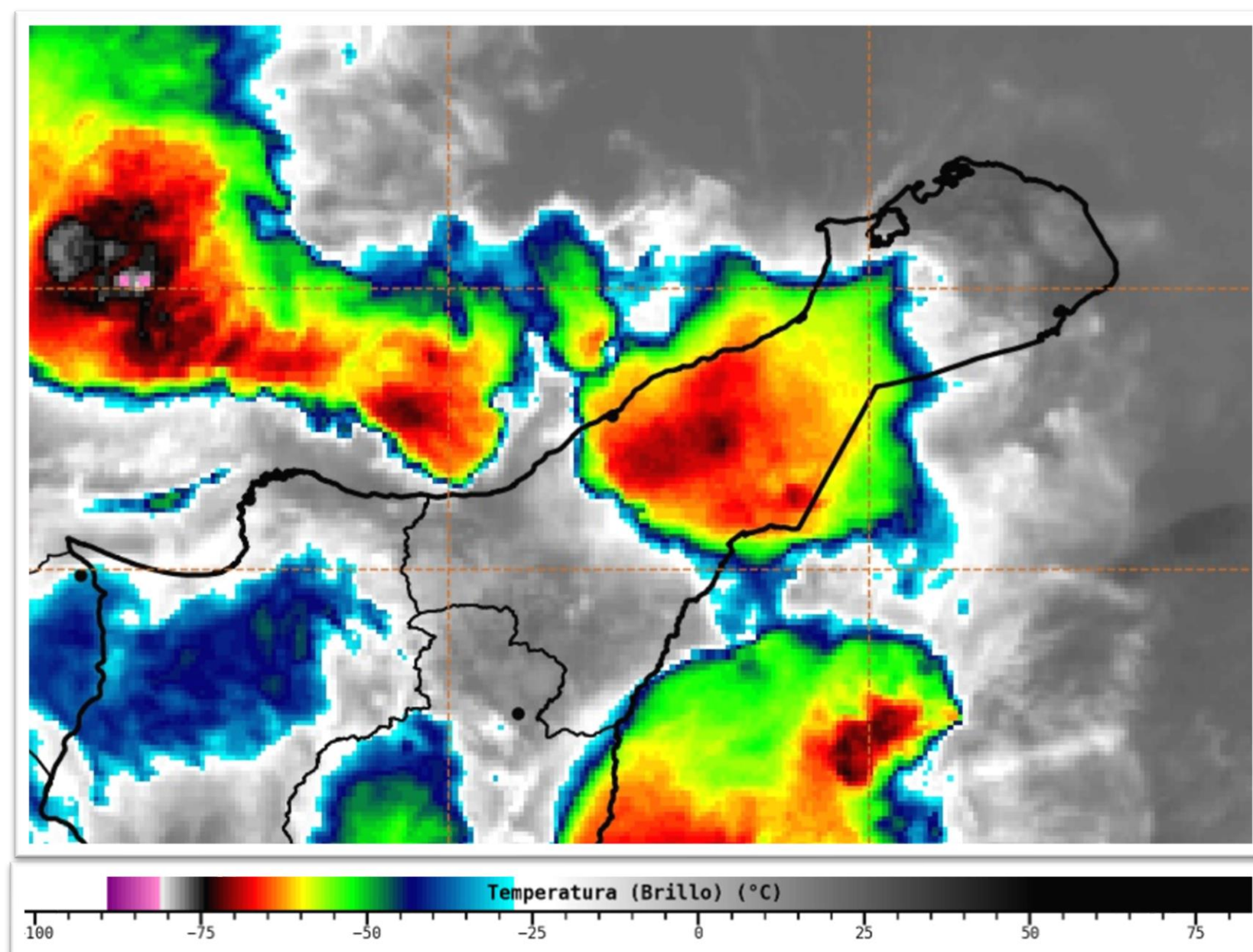
Imagen satelital Infrarojo GOES 16 Septiembre 22 de 2021 – Hora 9:00 HLC. Fuente: IDEAM
