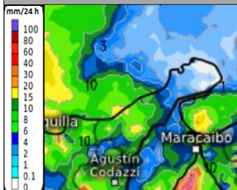
Pronóstico Precipitación Acumulada 24 horas Viernes 15 octubre
