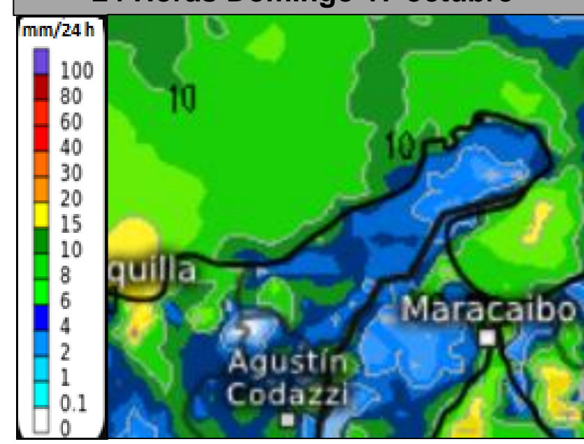
Pronóstico Precipitación Acumulada 24 Horas Domingo 17 octubre
