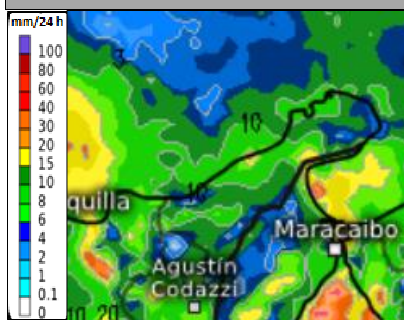
Pronóstico Precipitación Acumulada 24 horas Sábado 16 octubre
