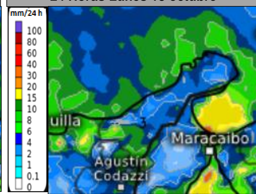
Pronóstico Precipitación Acumulada 24 Horas Lunes 18 octubre
