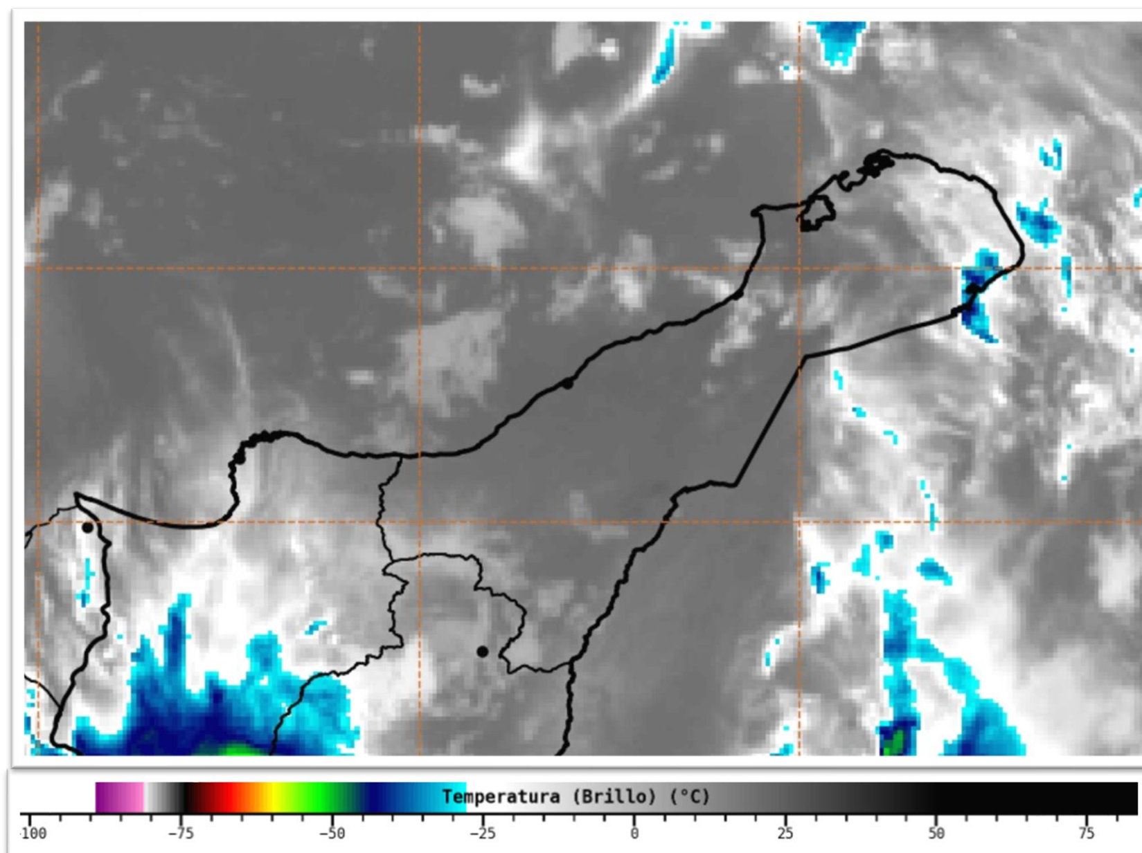
Imagen satelital Infrarojo GOES 16 Octubre 11 de 2021 – Hora 7:10 HLC. Fuente: IDEAM
