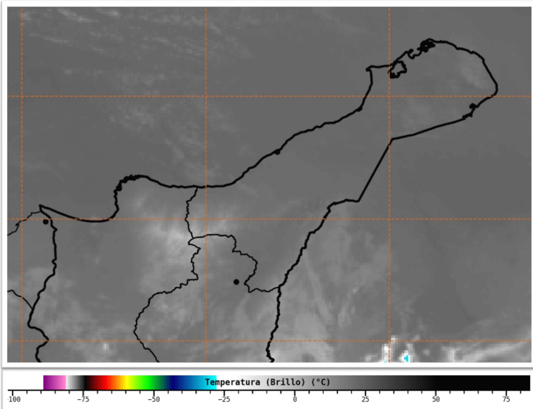
Imagen satelital Infrarojo GOES 16 Octubre 22 de 2021 – Hora 7:00 HLC. Fuente: IDEAM
