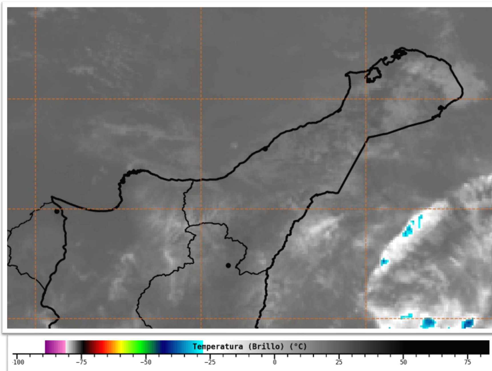
Imagen satelital Infrarojo GOES 16 Octubre 26 de 2021 – Hora 8:20 HLC. Fuente: IDEAM
