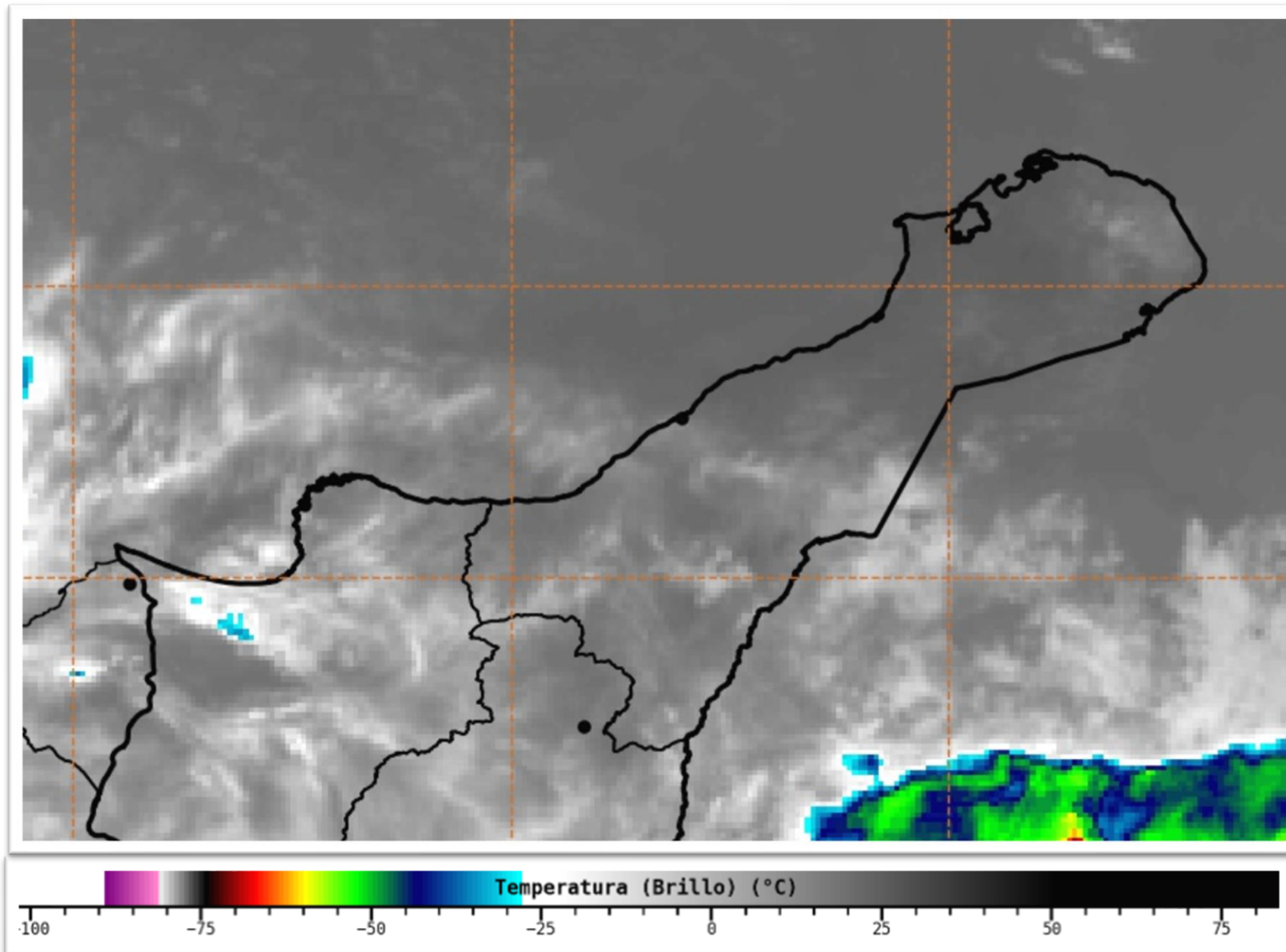
Imagen satelital Infrarojo GOES 16 Octubre 27 de 2021 – Hora 7:30 HLC. Fuente: IDEAM
