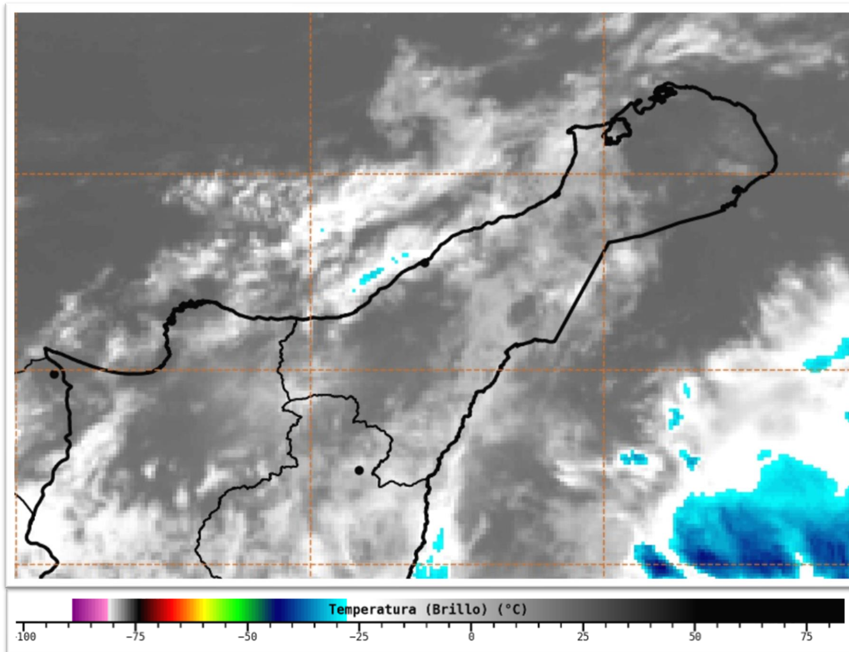
Imagen satelital Infrarojo GOES 16 Noviembre 02 de 2021 – Hora 7:20 HLC. Fuente: IDEAM
