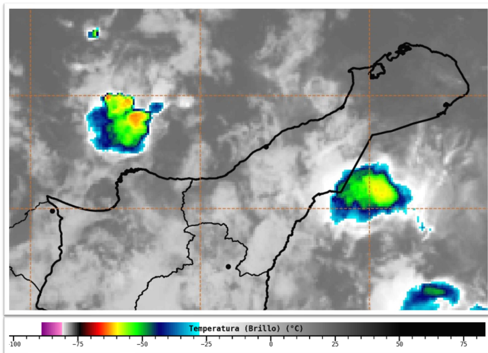
Imagen satelital Infrarojo GOES 16 Noviembre 04 de 2021 – Hora 7:20 HLC. Fuente: IDEAM
