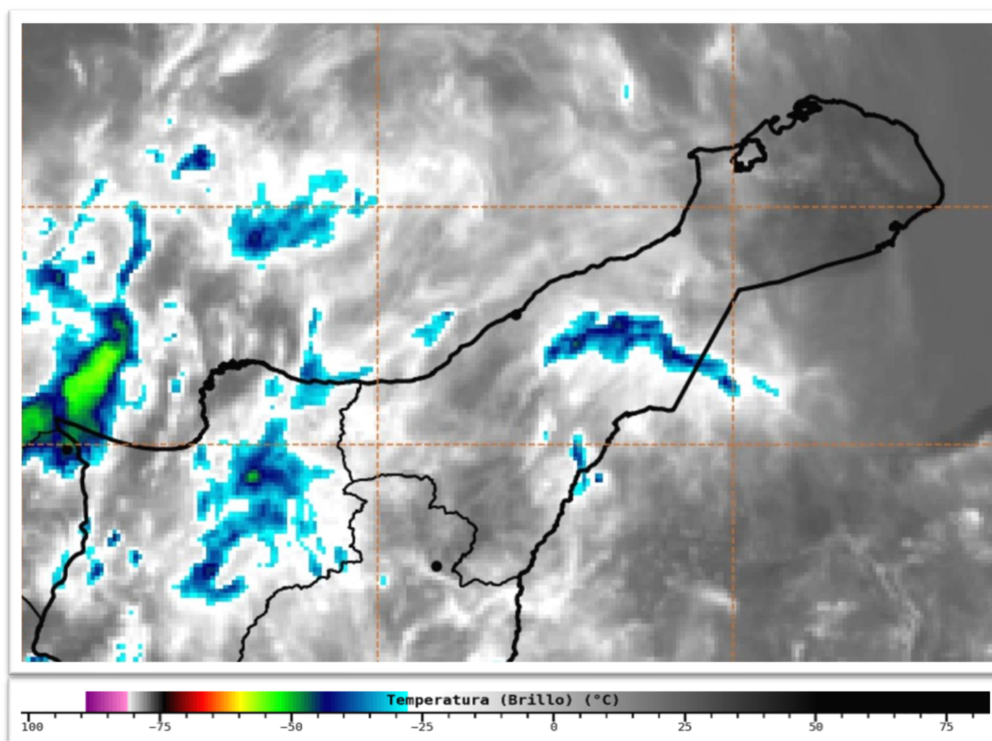
Imagen Satelital Infrarojo GOES 16 Noviembre 08 de 2021 – Hora 14:50 HLC. Fuente: IDEAM
