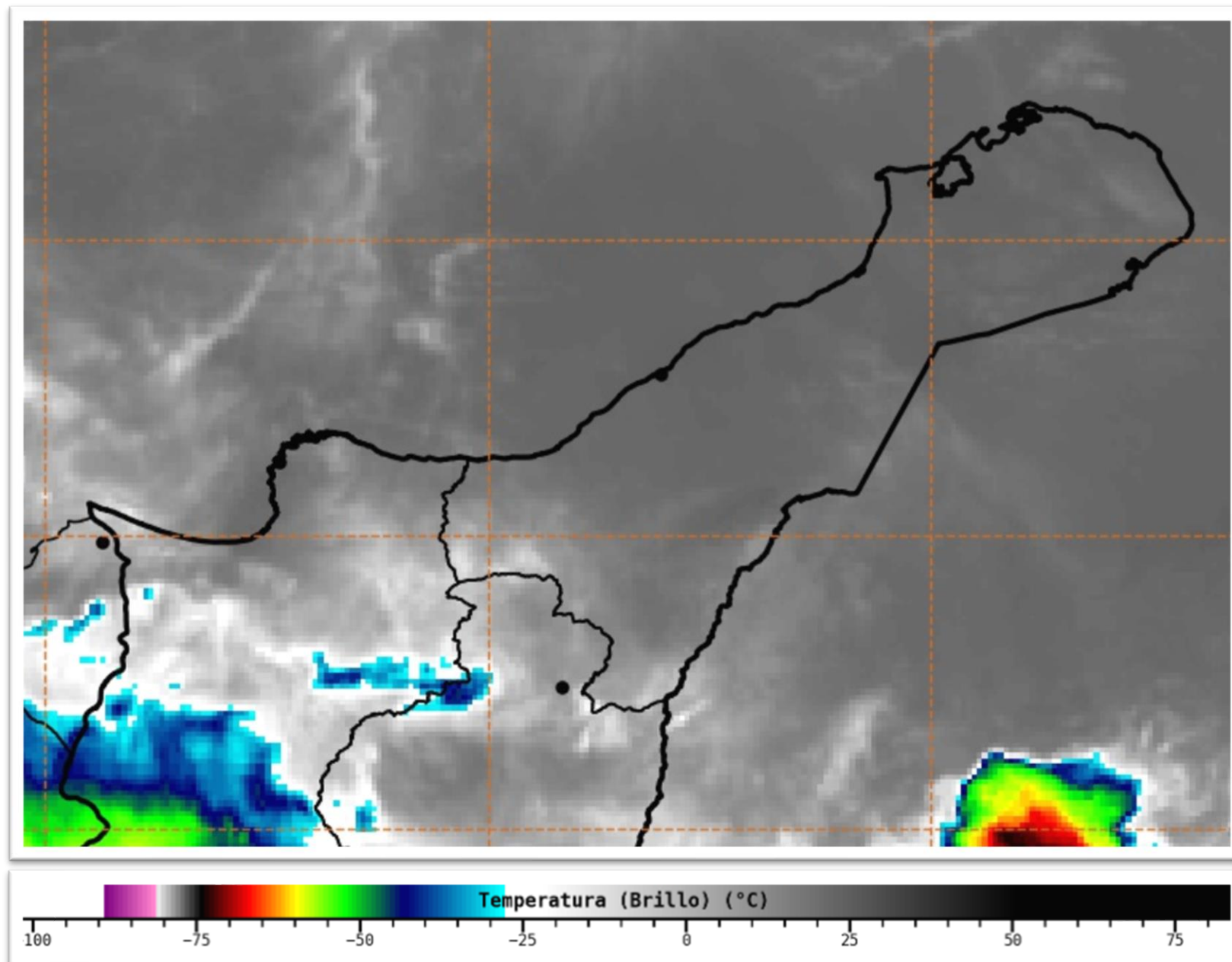
Imagen satelital Infrarojo GOES 16 Noviembre 08 de 2021 – Hora 7:20 HLC. Fuente: IDEAM
