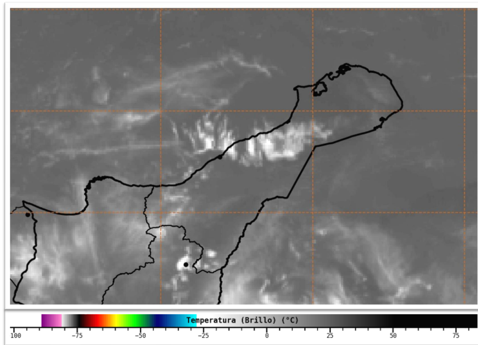
Imagen satelital Infrarojo GOES 16 Noviembre 09 de 2021 – Hora 7:20 HLC. Fuente: IDEAM
