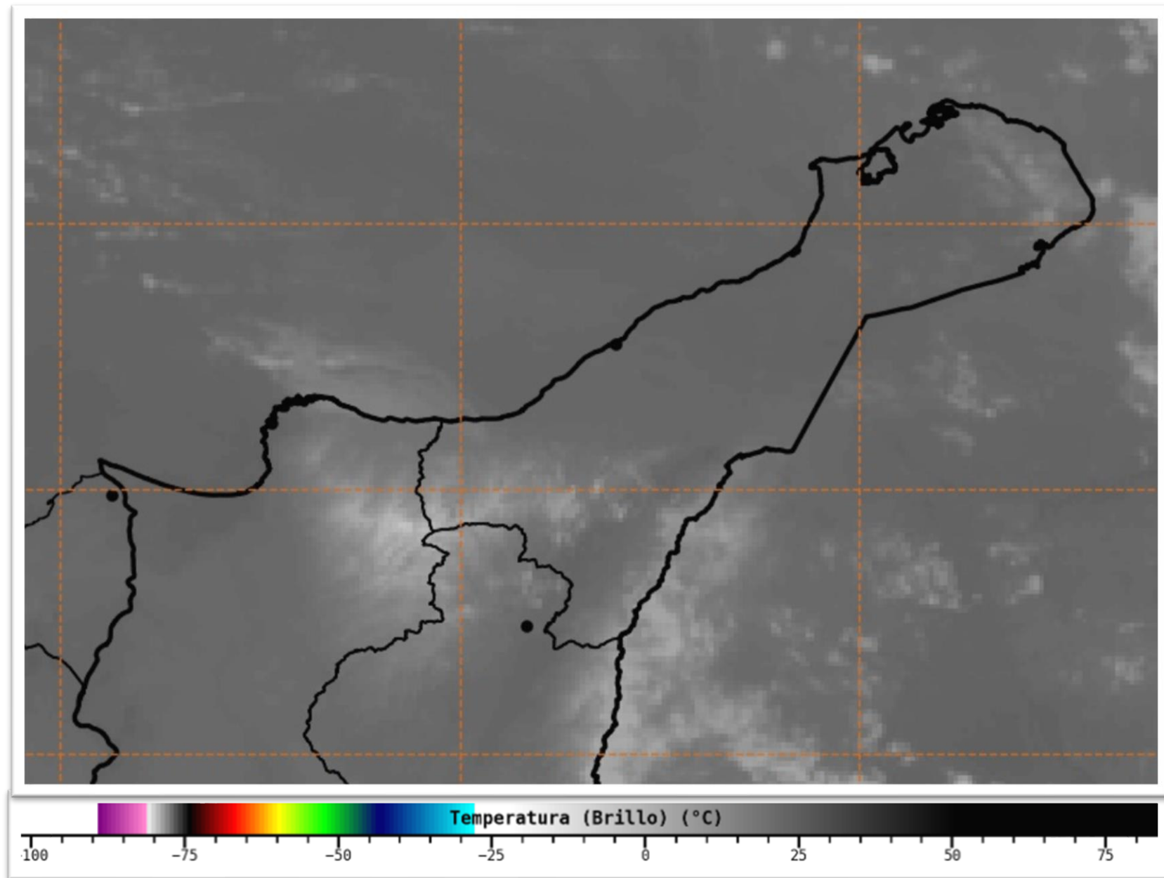
Imagen satelital Infrarojo GOES 16 Noviembre 12 de 2021 – Hora 7:20 HLC. Fuente: IDEAM
