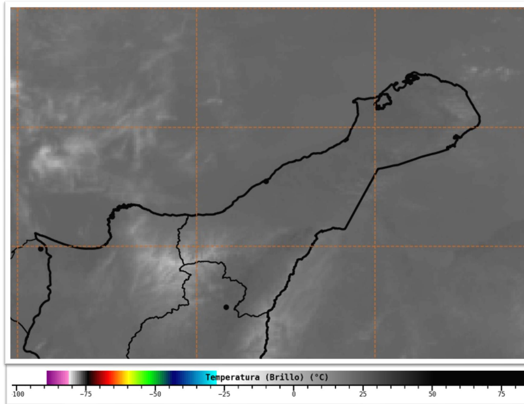
Imagen satelital Infrarojo GOES 16 Noviembre 18 de 2021 – Hora 7:30 HLC. Fuente: IDEAM
