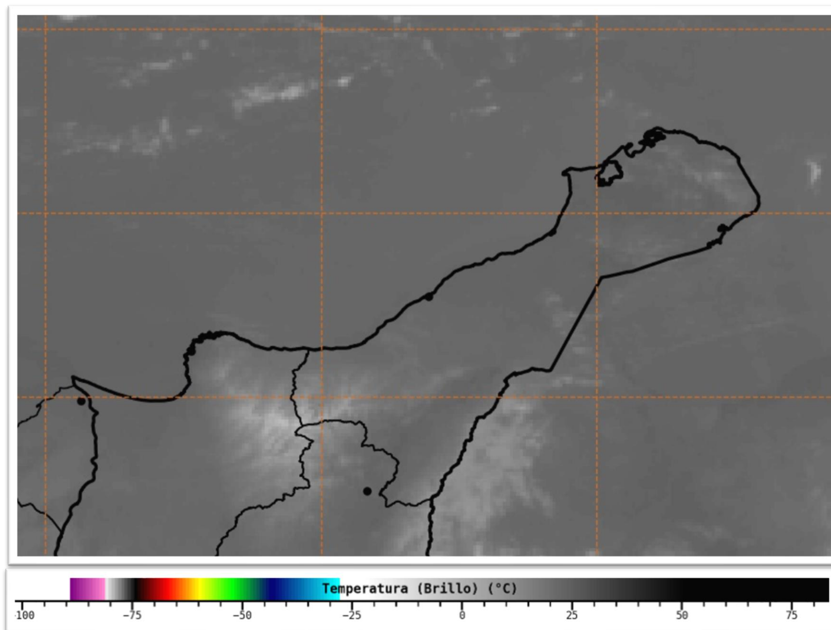
Imagen satelital Infrarojo GOES 16 Noviembre 19 de 2021 – Hora 7:30 HLC. Fuente: IDEAM
