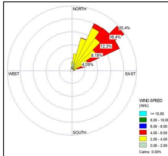
Figura 9. Rosa del Viento Horaria en diciembre de 2021.
