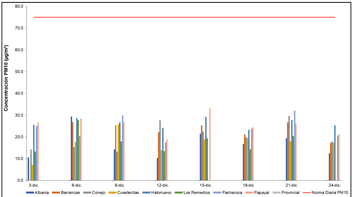
Figura 3. Comportamiento diario del PM10 en diciembre de 2021.
