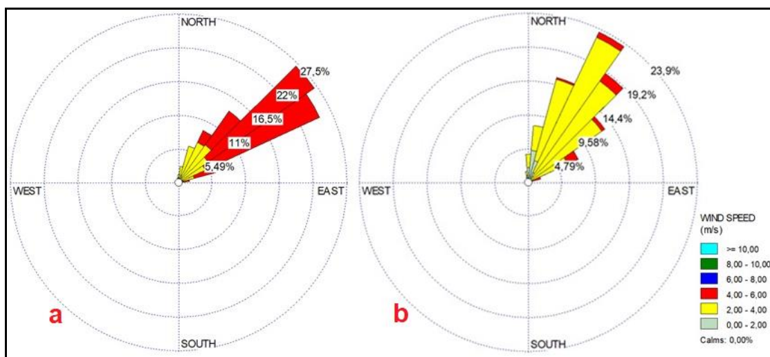
Figura 10. Rosa del Viento por periodo en diciembre de 2021. a) Diurno y b) Nocturno.
