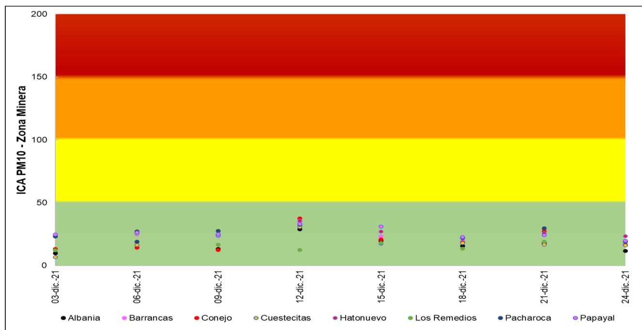
Figura 6. Índice de calidad del aire diario para el periodo evaluado.
