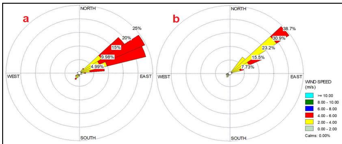
Figura 10. Rosa del Viento por periodo en abril de 2022. a) Diurno y b) Nocturno.
