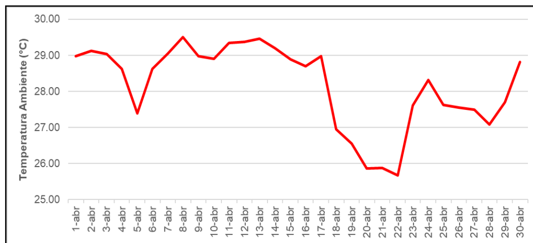
Figura 8. Comportamiento por día de la temperatura ambiente.
