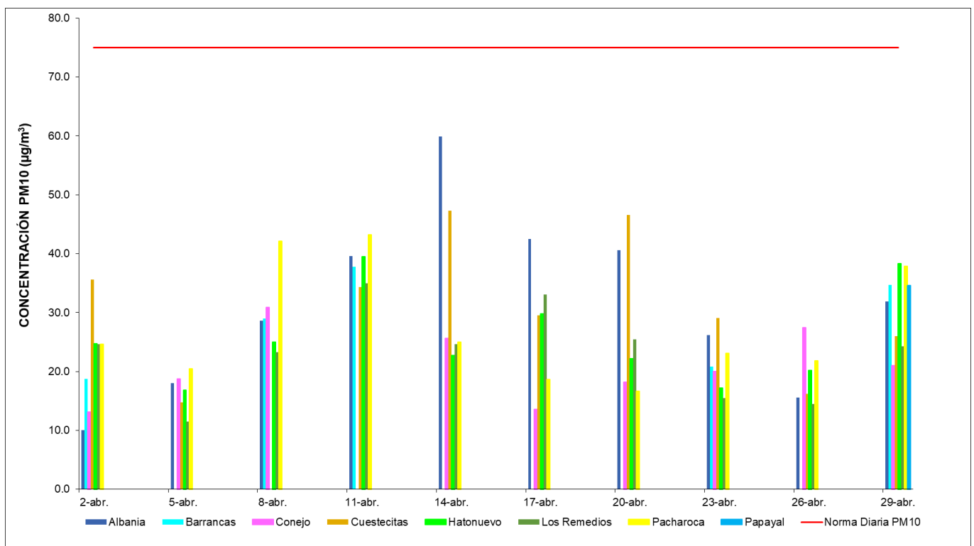
Figura 3. Comportamiento diario del PM10 en abril de 2022.
