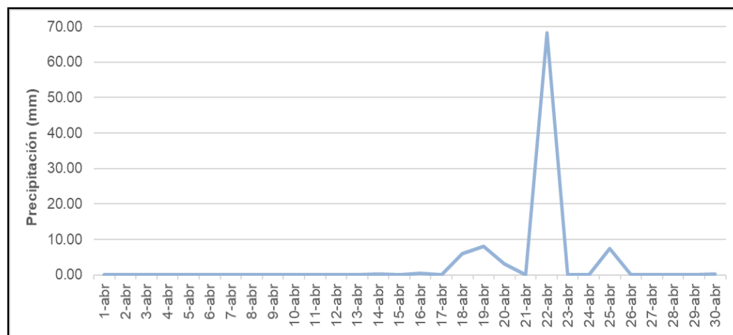
Figura 12. Precipitación diaria en abril de 2022.
