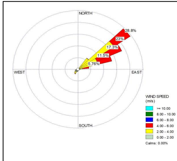
Figura 9. Rosa del Viento Horaria en abril de 2022.
