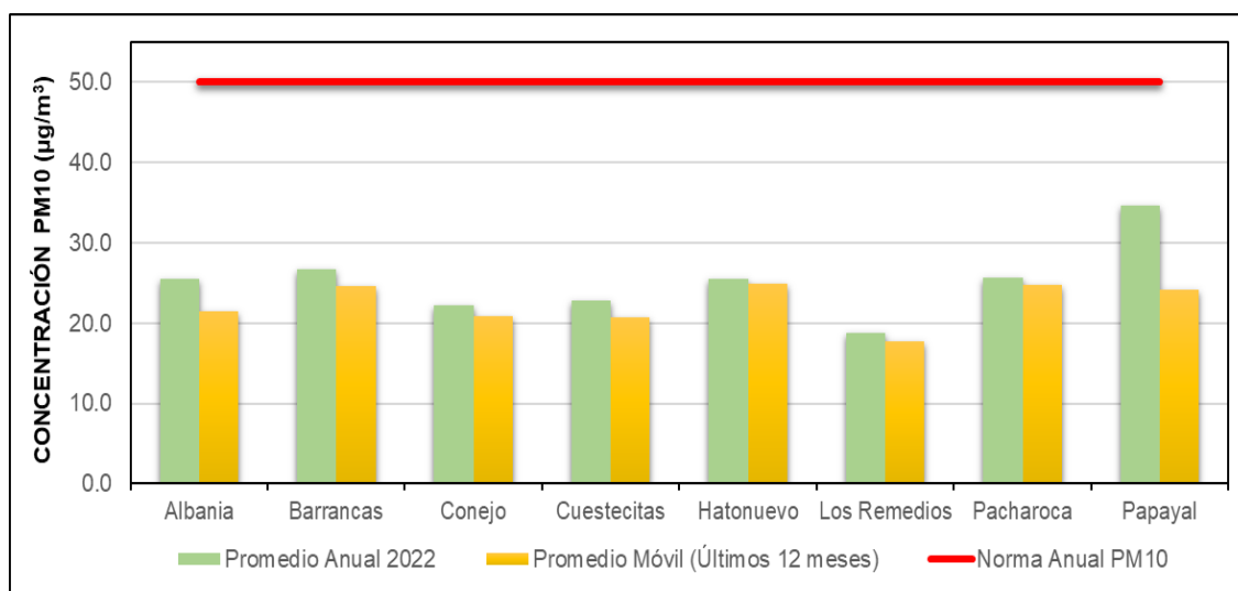
Figura 4. Promedio anual indicativo de PM10 para el SEVCA.
