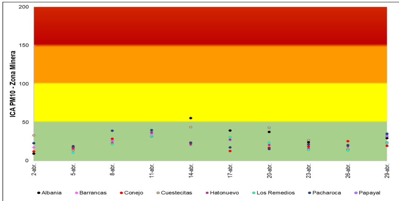
Figura 5. Índice de calidad del aire diario para el periodo evaluado.
