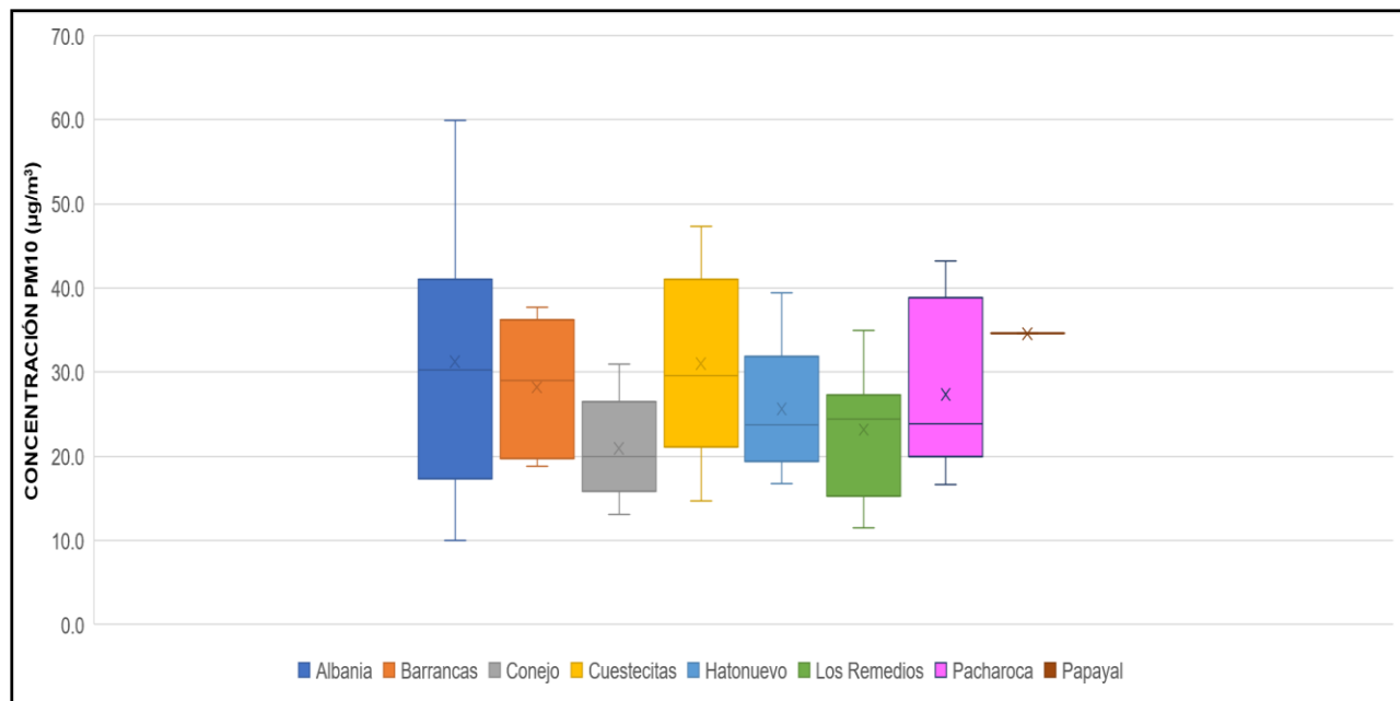
Figura 6. Dispersión de los datos en cada estación de monitoreo.
