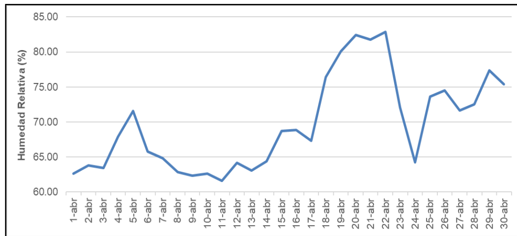
Figura 13. Humedad Relativa diaria en abril de 2022.
