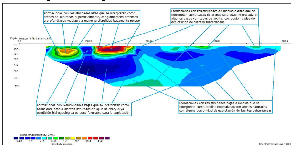
Figura 13. Geotomografía de resistividad No 3-7 método Wenner
