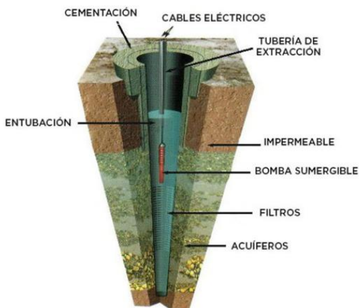
Figura 15. Consideraciones para la perforación
