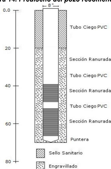
Figura 14. Prediseño del pozo recomendado
