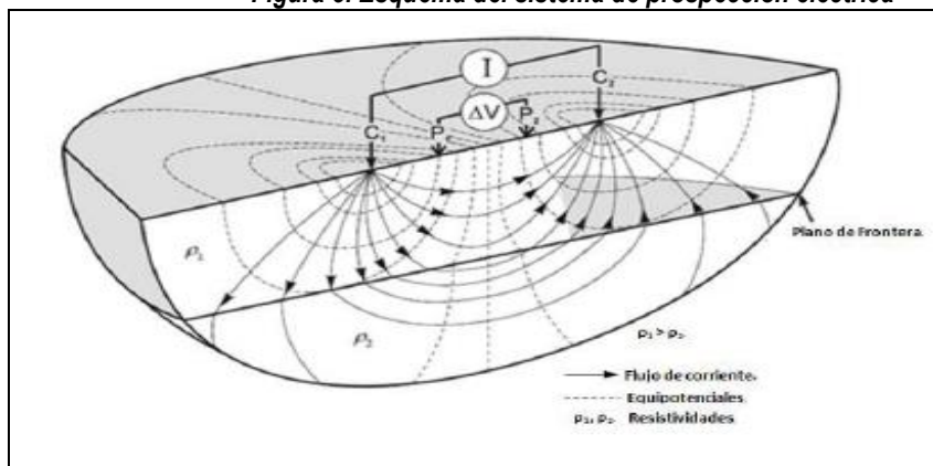
Figura 5. Esquema del sistema de prospección eléctrica
