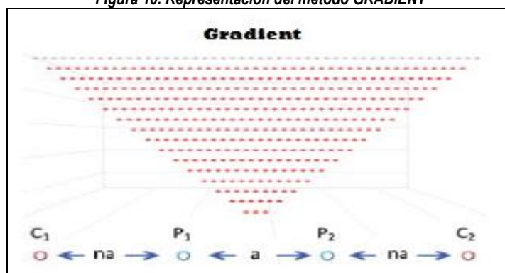
Figura 10. Representación del método GRADIENT
