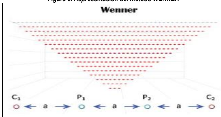
Figura 8. Representación del método WENNER
