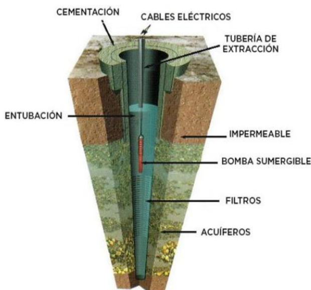
Figura 18. Consideraciones para la perforación
