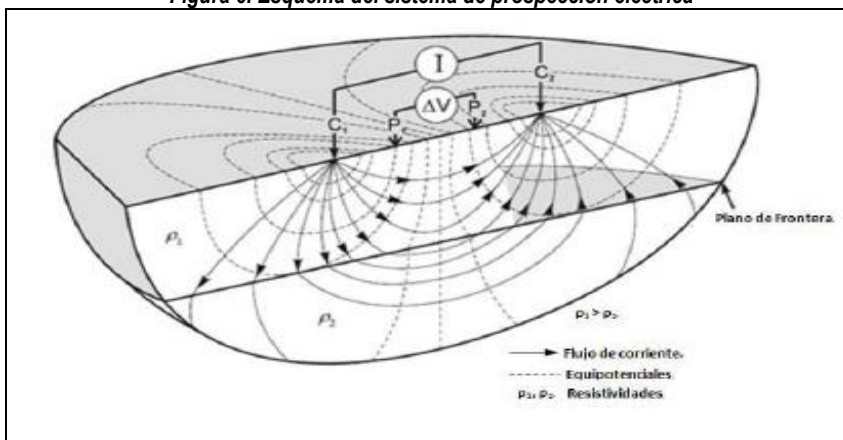
Figura 6. Esquema del sistema de prospección eléctrica
