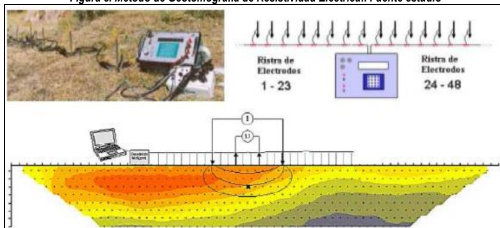
Figura 5. Método de Geotomografía de Resistividad Eléctrica.: Fuente estudio
