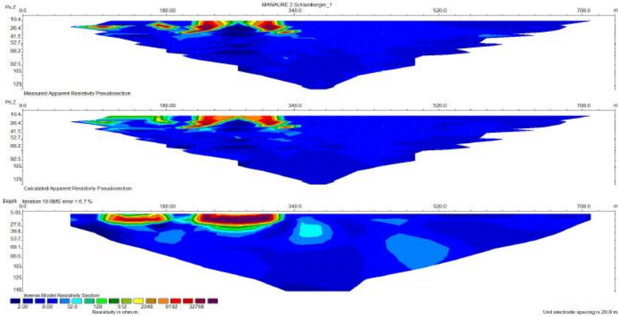
Figura 14. Geotomografía Modelo Gradient No. 2
