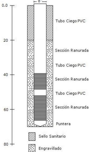
Figura 17. Prediseño del pozo recomendado
