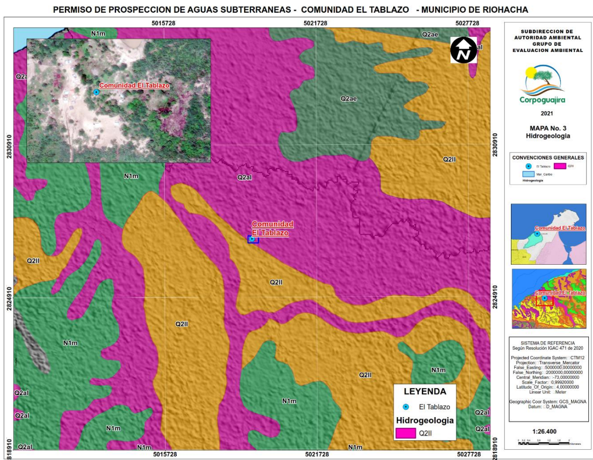
Figura 5. Hidrogeología
