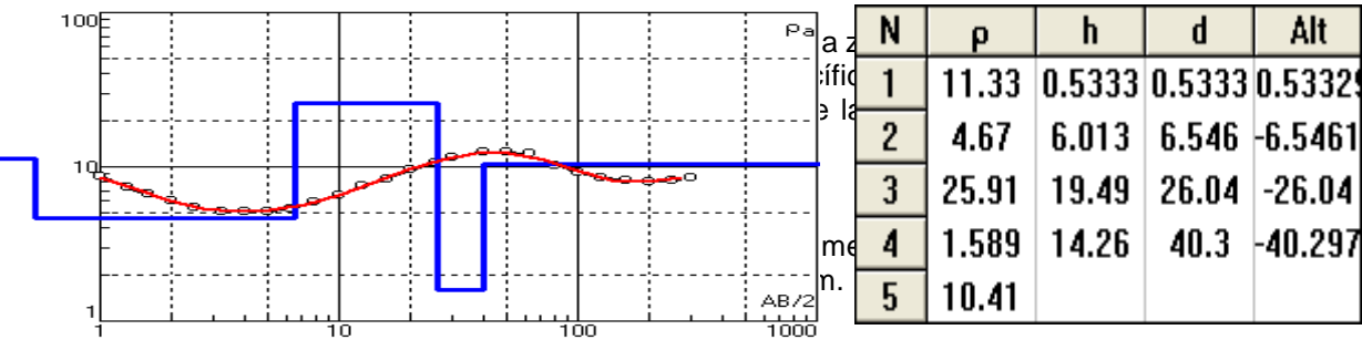
Figura 5. Curva teórica, datos y modelación para el sondeo SEV01.
